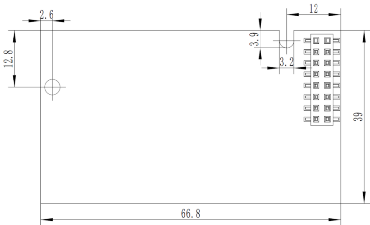
图1-2 KZ730-IO1卡外观尺寸
