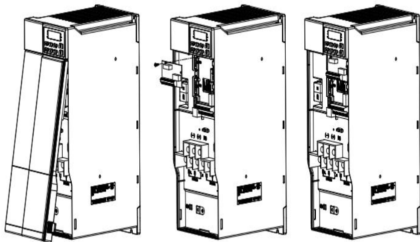
图2-1 KZ730-IO1卡安装示意图
