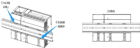
图 4. 1-1 导轨安装图
