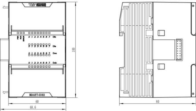
图 3. 3-1 MAST-D32 外观尺寸图
