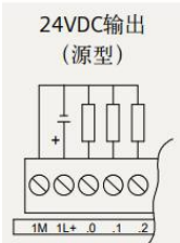
图 3. 5-2 普通 DO 输出外部接线图
