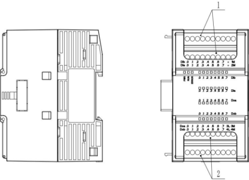
图 3. 1 MAST-D32 接口示意图
