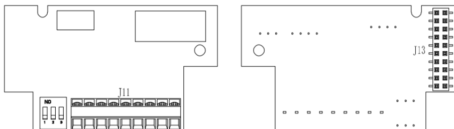
图1-3 KZ730-PG1卡接口布局
