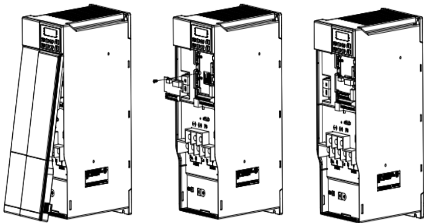
图2-1 KZ730-PG1卡安装示意图
