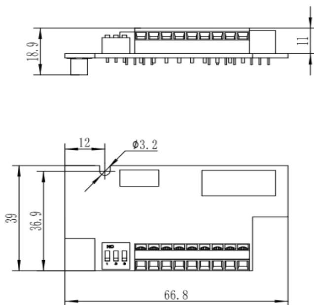
图1-2 KZ730-PG1卡外观尺寸
